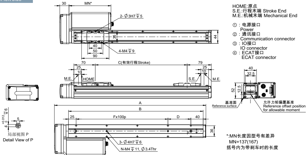
尺寸图代号说明 · 质量 Dimensions, Mass
